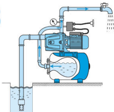
Рис.13 При возобновлении водоразбора, вода, находящаяся в гидроаккумуляторе под давлением, начинает поступать потребителю. Давление в системе при этом постепенно снижается, а насос остается выключенным
