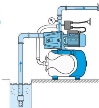
Рис.14 Когда давление воды в системе понижается до настроенного уровня - давления включения , реле включает насос
