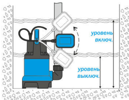
рис. 6а - автоматический режим
